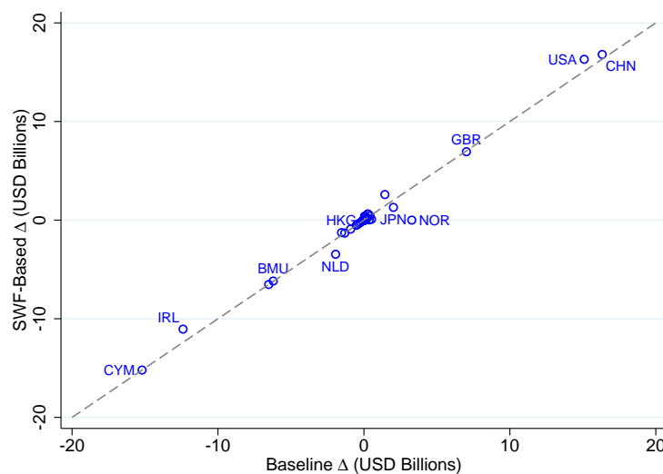
(d) Norway, Equities: Funds vs. SWF
